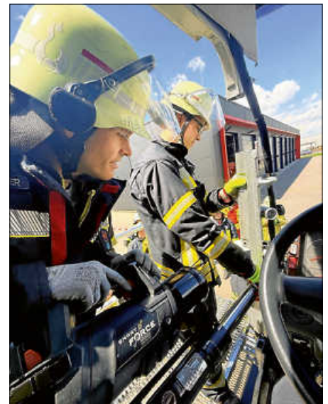
Station: Technische Hilfeleistung an LKW Foto: Feuerwehr Bad Saulgau
